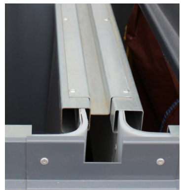
Kuva 3. U-listan kiinnitys
