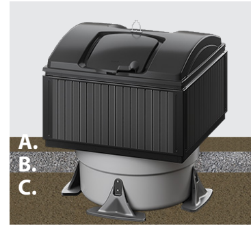
Kuva 2. Kuopan täyttäminen A. Viimeistelykerros, 100 mm B. Ankkurointikerros, sepeli 0/32, 400 mm C. Tasekerros, murske 0/16, väh. 50 mm
