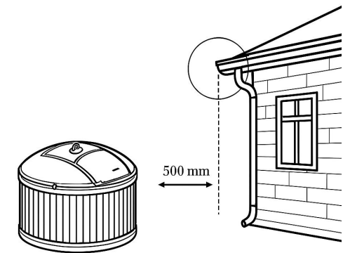
Kuva 2. Etäisyys räystääseen
